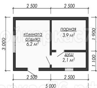
План 1-го этажа
