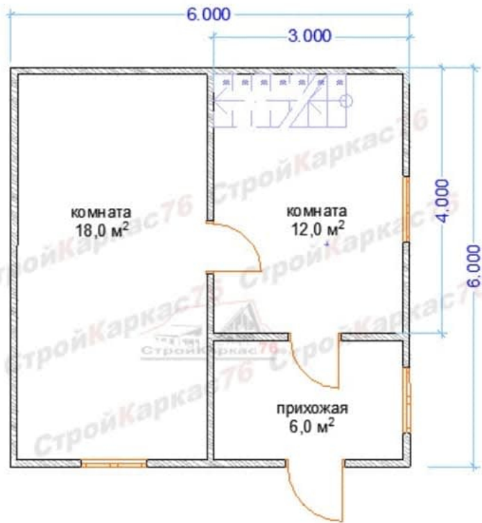
План 1-ого этажа
