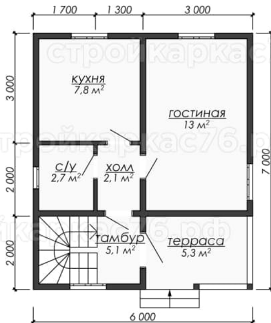
План 1-го этажа
