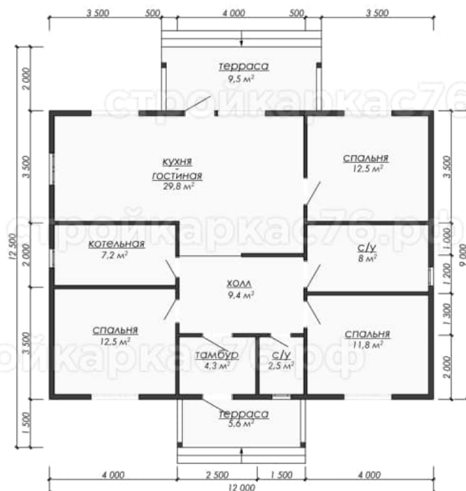
План 1-го этажа
