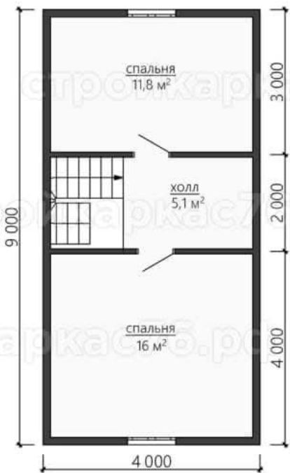
План 2-го этажа
