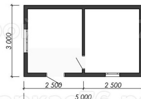
План 1-го этажа
