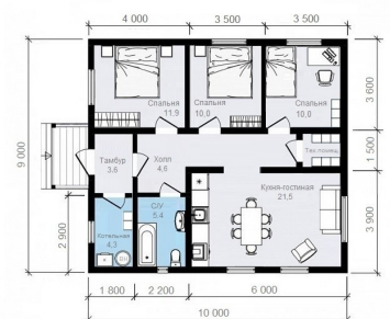
План 1 этажа
