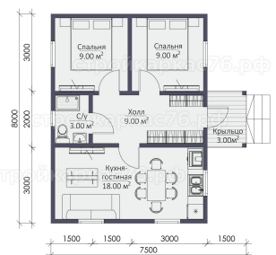
План 1 этажа
