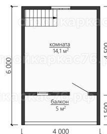
План 1-го этажа
