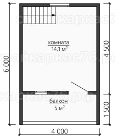
План 1-го этажа
