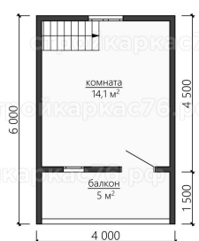
План 2-го этажа
