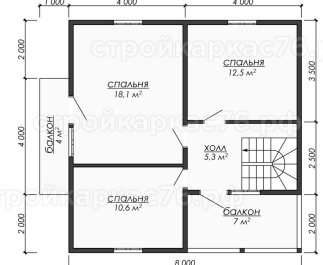
План 2-го этажа
