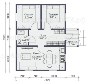
План 1 этажа
