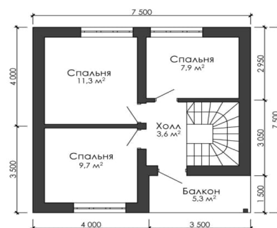
План 2-го этажа
