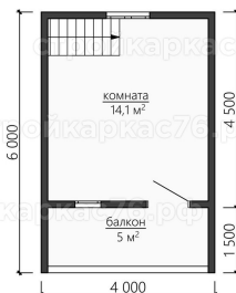
План 1-го этажа
