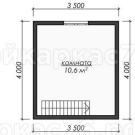
План 2-го этажа
