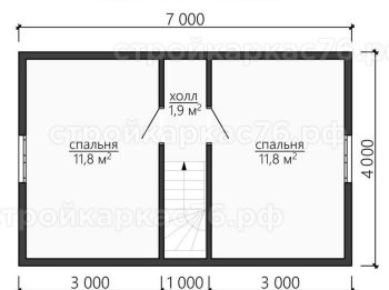
План 2-го этажа
