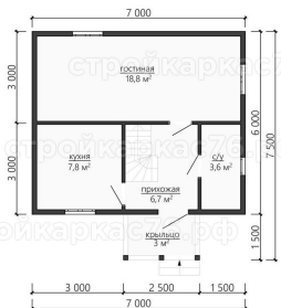
План 1-го этажа
