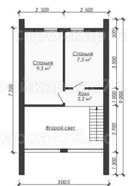
План 2-го этажа
